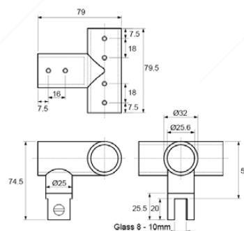
GLASS HOLDER GH 25-04 CP
