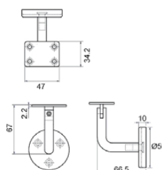
SCH 0312 RW STRAIGHT SSS Available: SCH 0312 RW OVAL SSS
